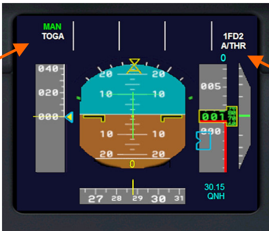
Image 56 – Mode TOGA en décollage manuel.
